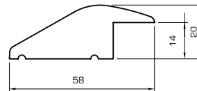
Winkelleiste
